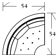
ITEM # 20-545 Wedge 54 x 54 x 33 SW: 50 SD: 25 SH: 17
